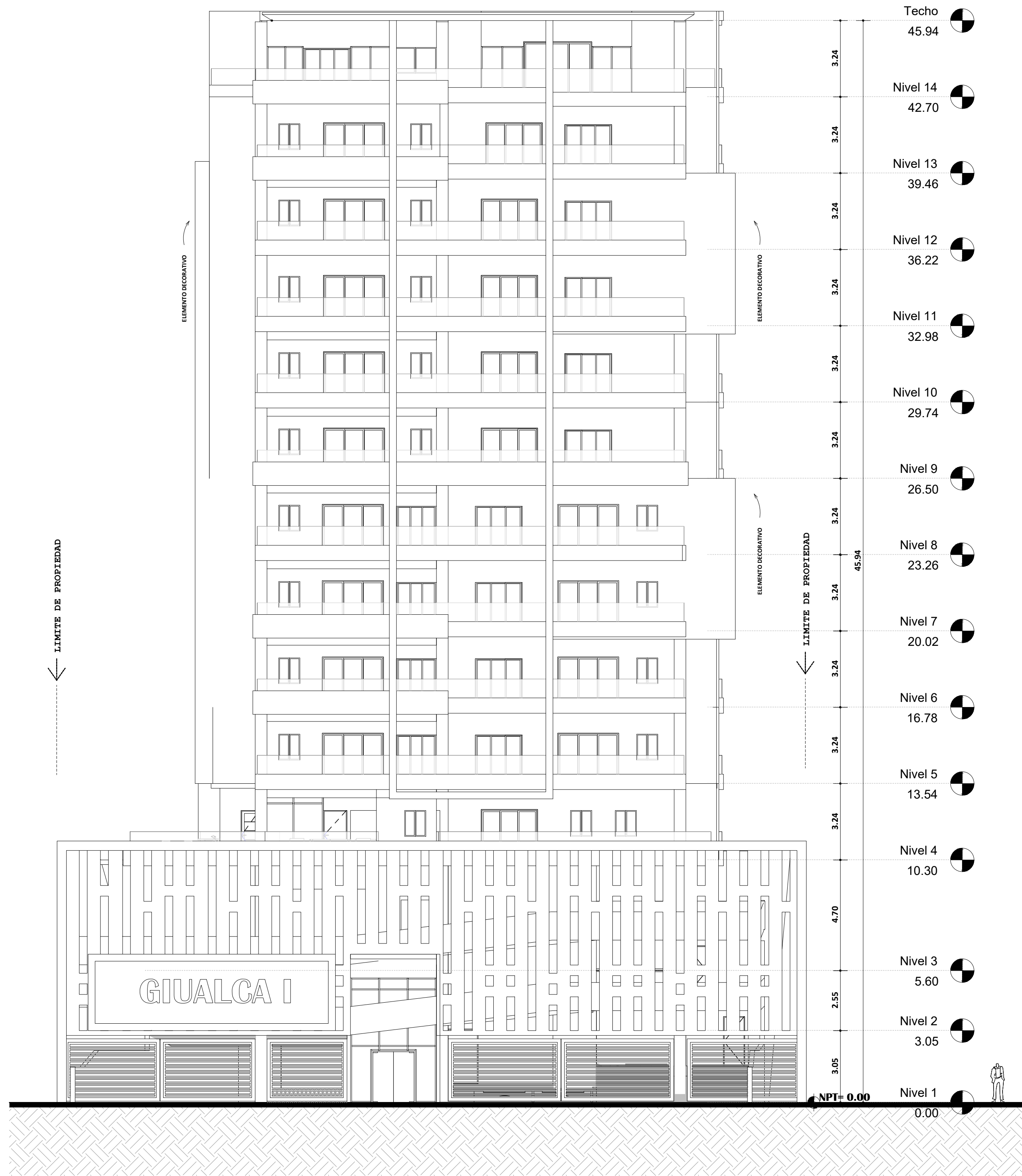
ELEVACION FRONTAL
