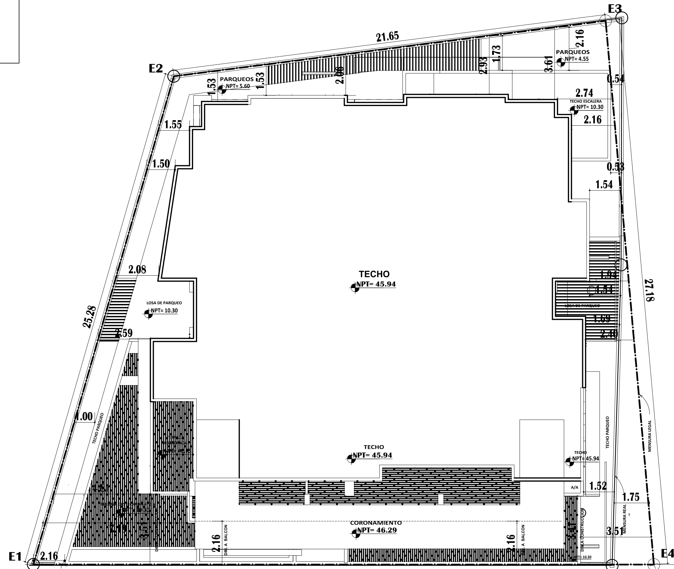
PLANTA DE SUPERPOSICION DE SOLARES CON LINDEROS
