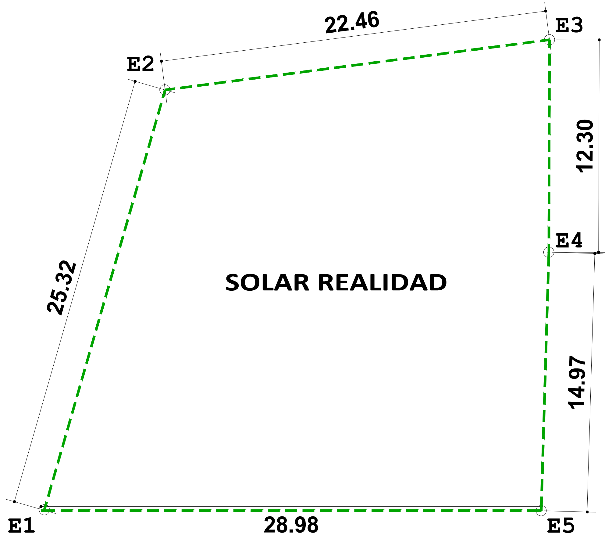
MENSURA DE LEVANTAMIENTO REAL
