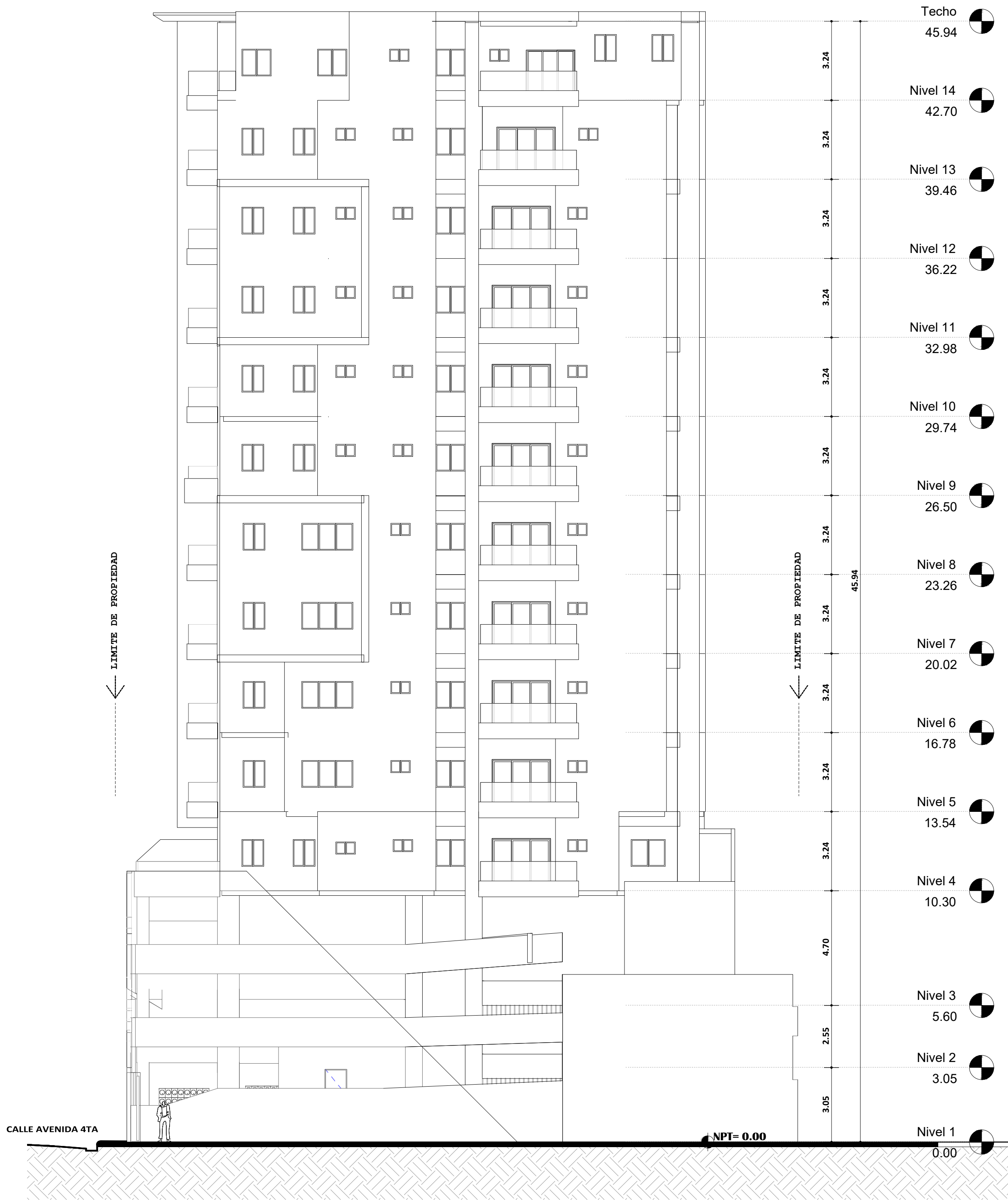
ELEVACION LATERAL DERECHA
