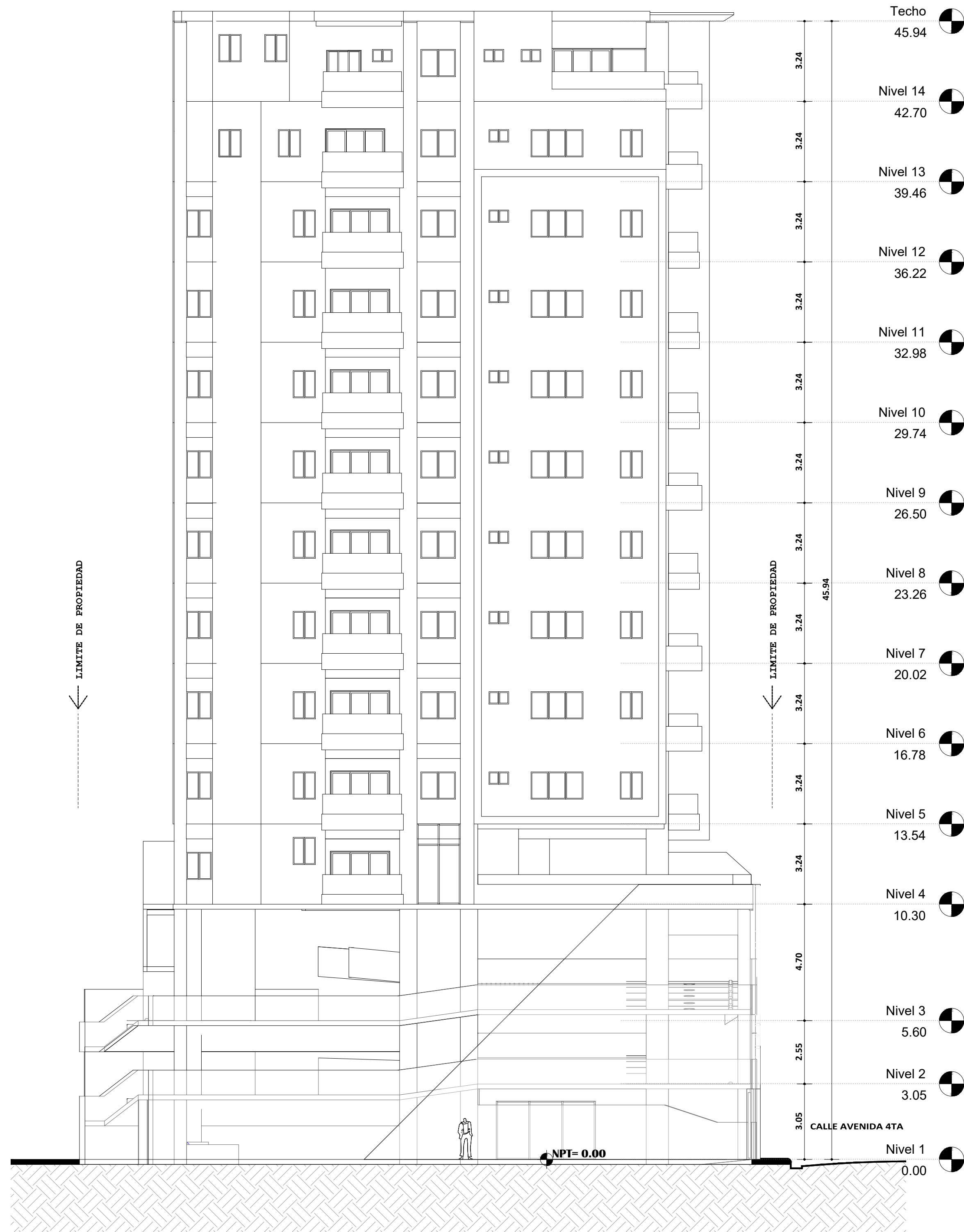
ELEVACION LATERAL IZQUIERDA
