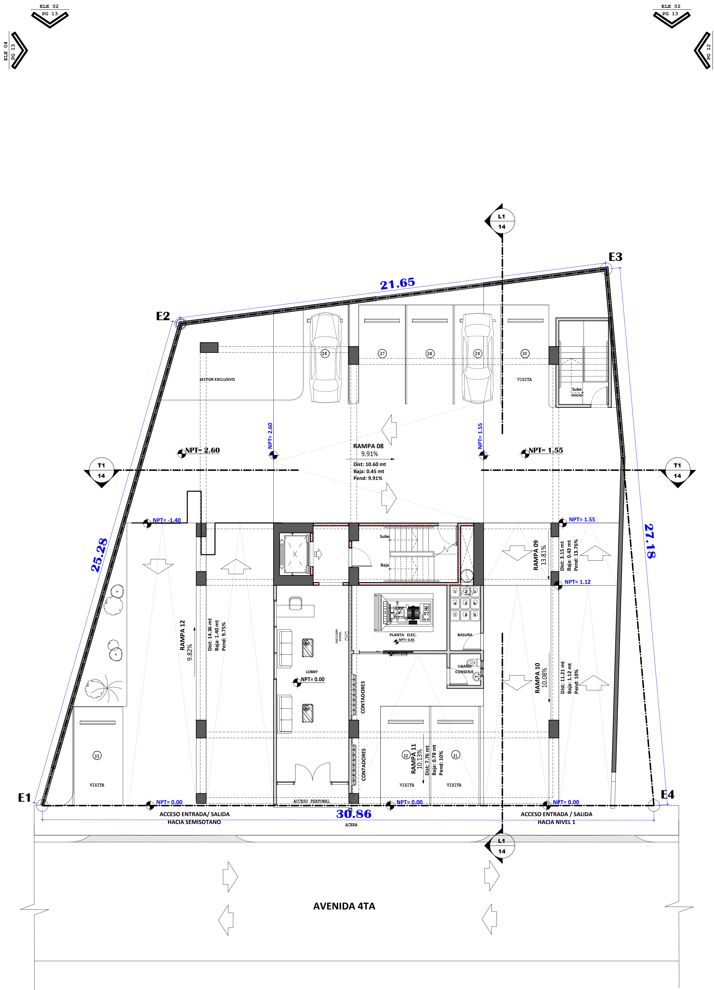
PLANTA ARQ. AMUEBLADA NIVEL 1
