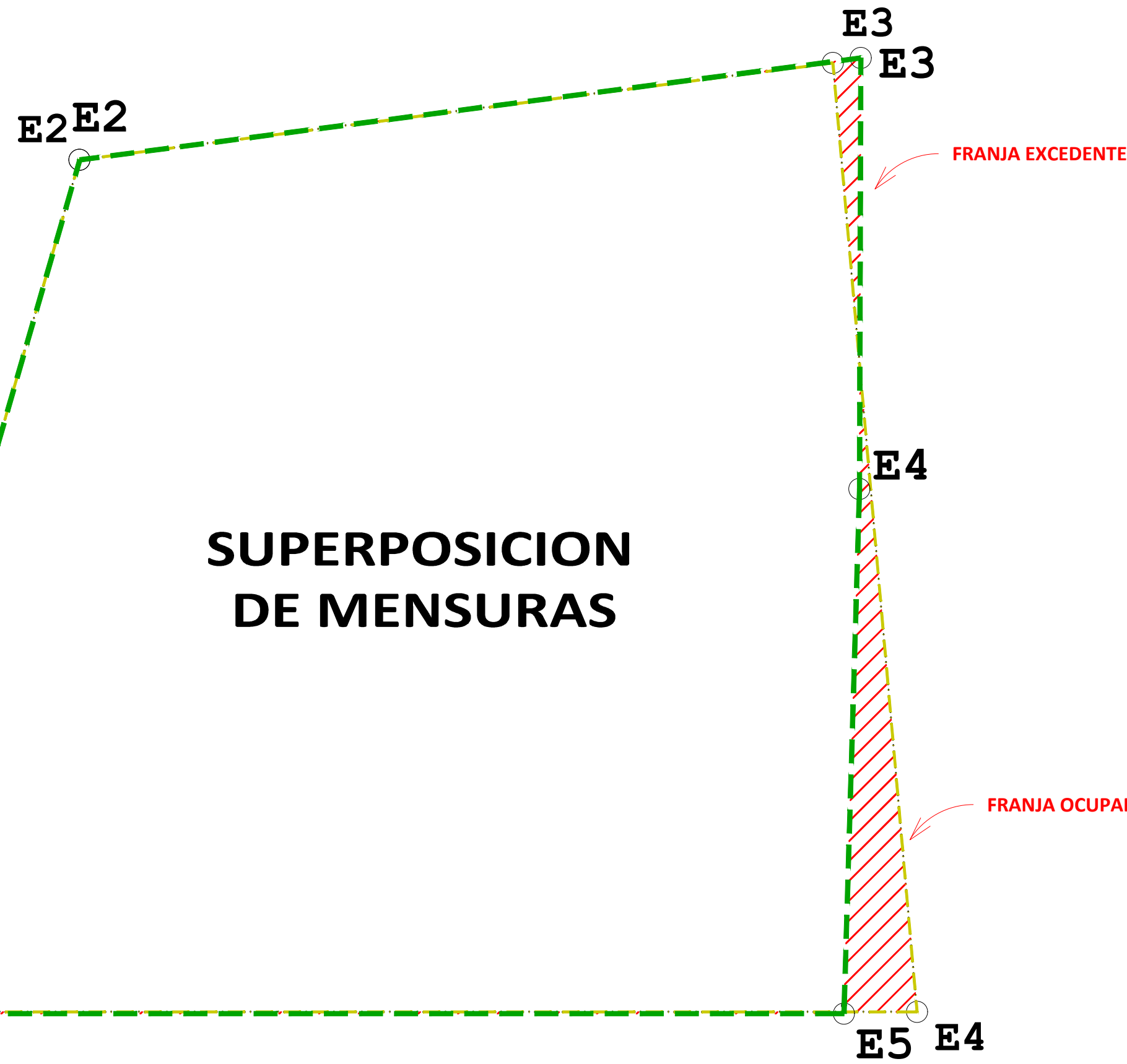
MENSURA CATASTRAL LEGAL + LEVANTAMIENTO REAL
